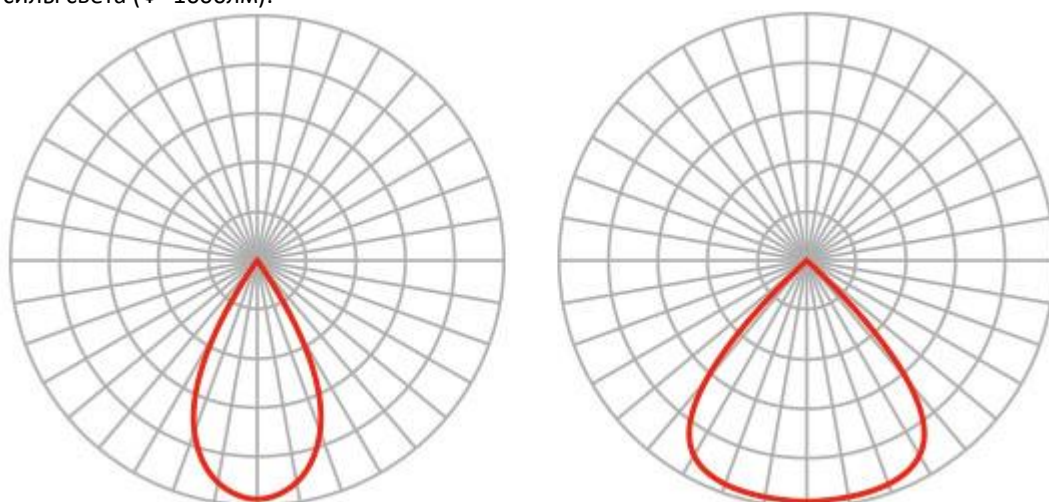
Рисунок 2. Кривые силы света
