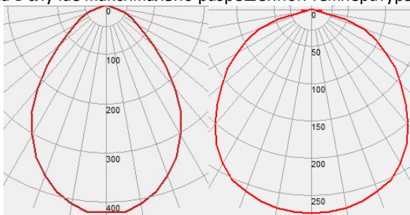
Рисунок 2. Кривые силы света для светильника с углом обзора 2Q_{1/2}=70 и 120 соответственно
